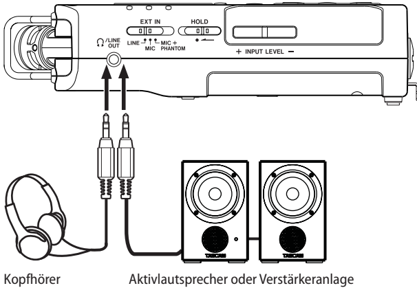
Kopfhörer
