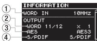
[リファレンスリダナント機能がオンのときの表示例]
